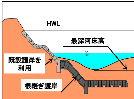
図 5-13 根継ぎ護岸イメージ
